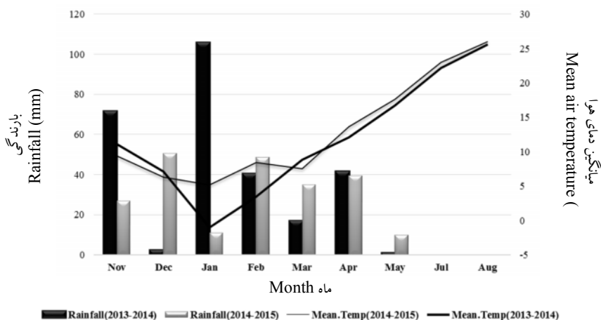
شکل ۱- میانگین دما و بارش کل ماهانه در طول فصل رشد در ایستگاه باجگاه فارس، شیراز (۱۳۹۲-۹۳ و ۱۳۹۳-۹۴)
