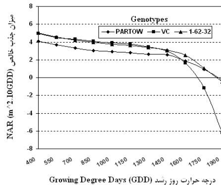
شکل ۱۱- تغییرات میزان جذب خالص در ژنوتیپ‌های ماش Fig. 11. Variation in Net Assimilation Rate in Mungbean genotypes
