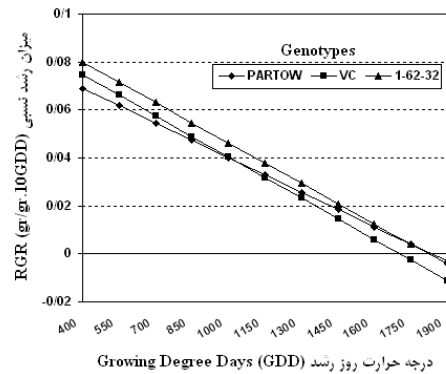
شکل ۷- تغییرات میزان رشد نسبی در ژنوتیپ‌های ماش Fig. 7. Variation in Relative Growth Rate in Mungbean genotypes
