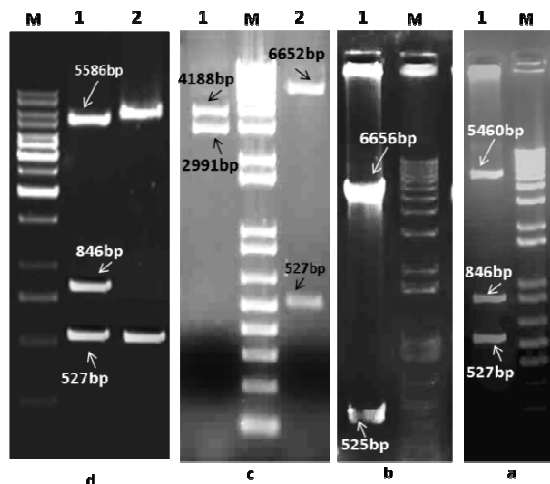
شکل ۳- آنالیز هضم آنزیمی با آنزیم HindIII ، به منظور آنالیز حضور و صحت قطعه FR در حامل های اختصاصی پلاستییدی ساخته شده برای گیاهان توتون، ذرت، کاهو، کلزا و گوجه فرنگی
