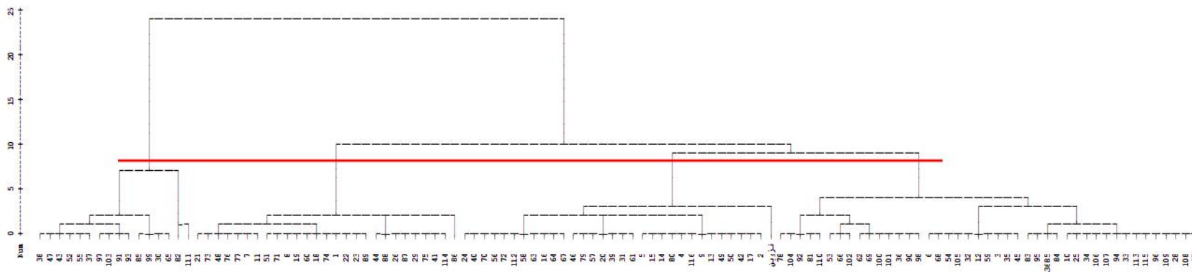
شکل ۱- دندروگرام حاصل از تجزیه خوشه‌ای صفات زراعی در لاین‌های خالص نوترکیب عدس (میانگین ۱۳۹۱ و ۱۳۹۲)
