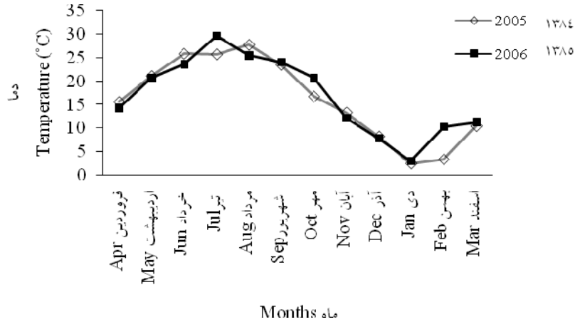
شکل ۱- میانگین دمای ماهانه دو سال ۱۳۸۴ و ۱۳۸۵
