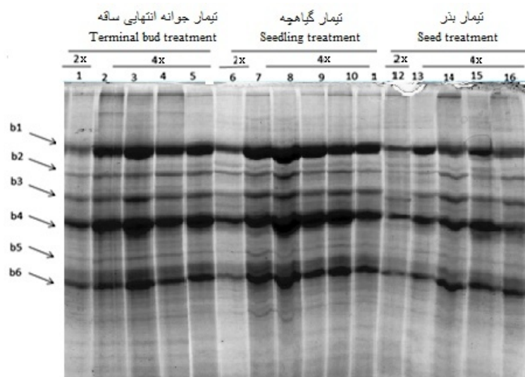
شکل ۲- تغییرات سطح بیان پروتئین‌های کل محلول در برگ‌های گیاه سورگوم در گیاهان تتراپلوئید و دیپلوئید، در سه روش تیمار با کلشسی‌سین
