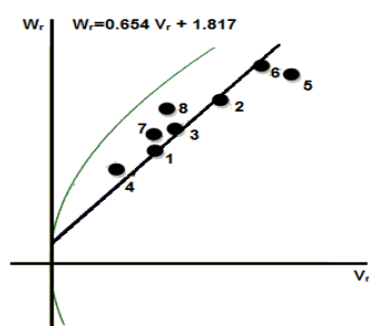
شکل ۶- رگرسیون W_r روی V_r برای صفت طول خوشه ژنوتیپ‌های برنج (۱: دیلمانی، ۲: طارم محلی، ۳: IR18430-46، ۴: لاین ۲۳، ۵: IR50، ۶: RI18442-1، ۷: RI18447-2، ۸: گیلانہ)
