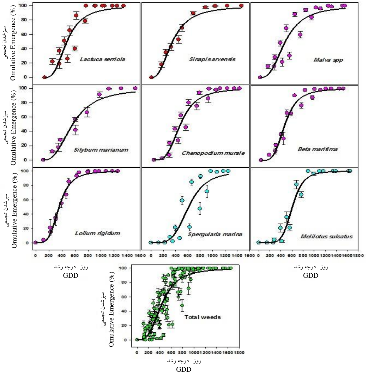
شکل ۱- مقادیر مشاهده شده (علامت‌ها) و پیش‌بینی شده (خطوط) رویش تجمعی علف‌های هرز در مزرعه کلزا با استفاده از معادله هیل
