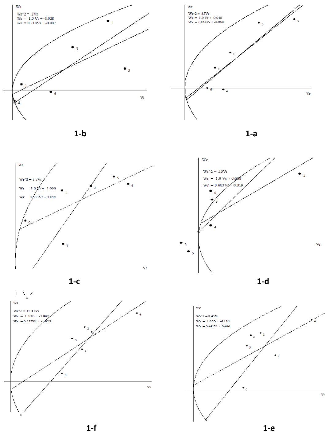
شکل ۱- رگرسیون Wr بر روی Vr برای صفات گیاهی مورد مطالعه و موقعیت ژنوتیپ‌های والدینی برنج از حیث توزیع و درجه غالبیت ژن‌ها، ۱: طارم، ۲: غریب، ۳: شاه پسند، ۴: درفک، ۵: سپیدرود و ۶: IR28 می‌باشند، و 1-a: محتوای سدیم، 1-b: میزان ماده خشک، 1-c: شاخص تحمل شوری، 1-d: روز تا گلدهی، 1-e: دانه در خوشه و 1-f: ارتفاع بوته می‌باشند
